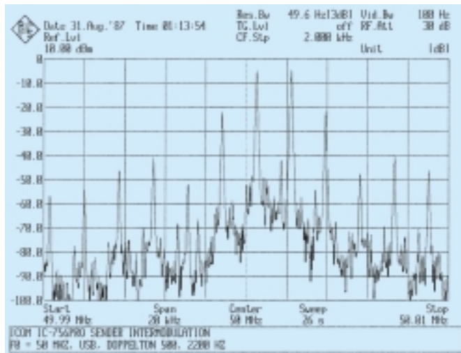
Bild S4: Sender-Intermodulation (6 m)
