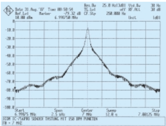
S7: Clickspektrum (Tastverhalten) bei CW (identisch für KW und 6 m)
