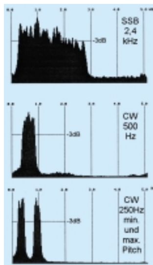
Bild E11: NF-Frequenzgang
