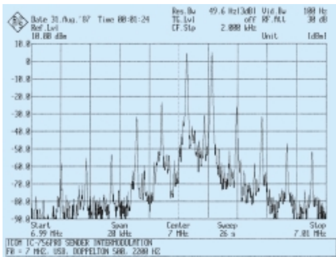
Bild S4: Sender-Intermodulation (KW)
