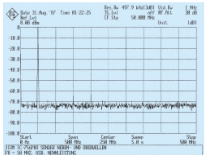
Bild S3: Sender-Neben- und Oberwellen (6 m)
