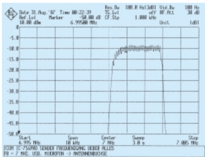
Bild S6: Sender-Frequenzgang (KW und 6 m)
