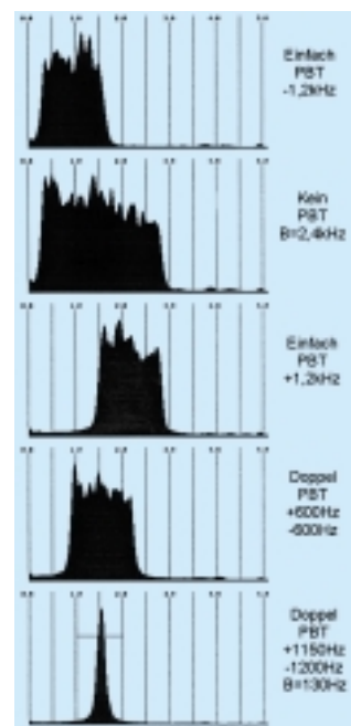
Bild E11: Passbandtuning
